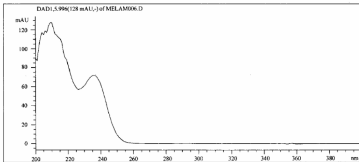
图 A.2 三聚氰胺紫外光谱图
