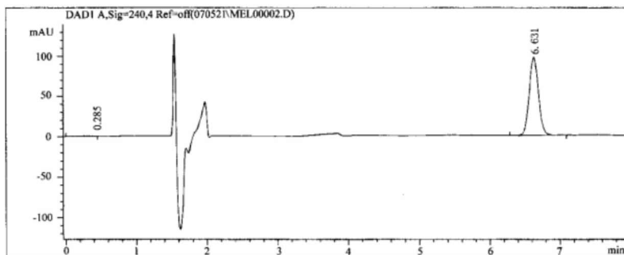
图 A.1 三聚氰胺标准色谱图
