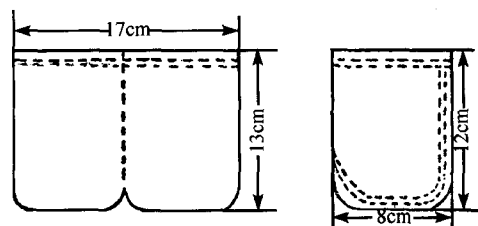
图 E.1 实验用袋的尺寸
