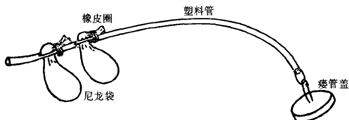
图 E.2 尼龙袋固定图示
