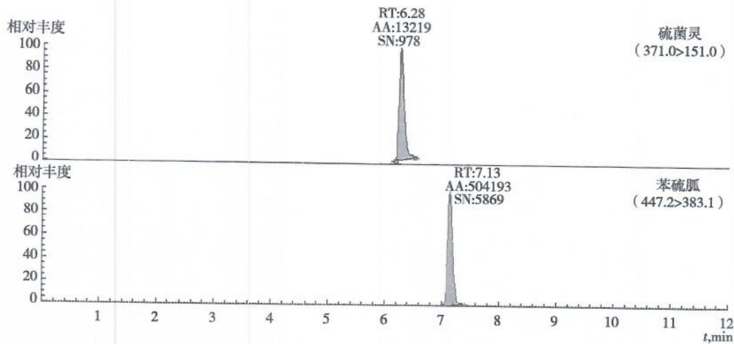
图 A. 1 苯硫脲和硫菌灵标准溶液(0.001 \mu\text{g/mL} )定量离子色谱图
