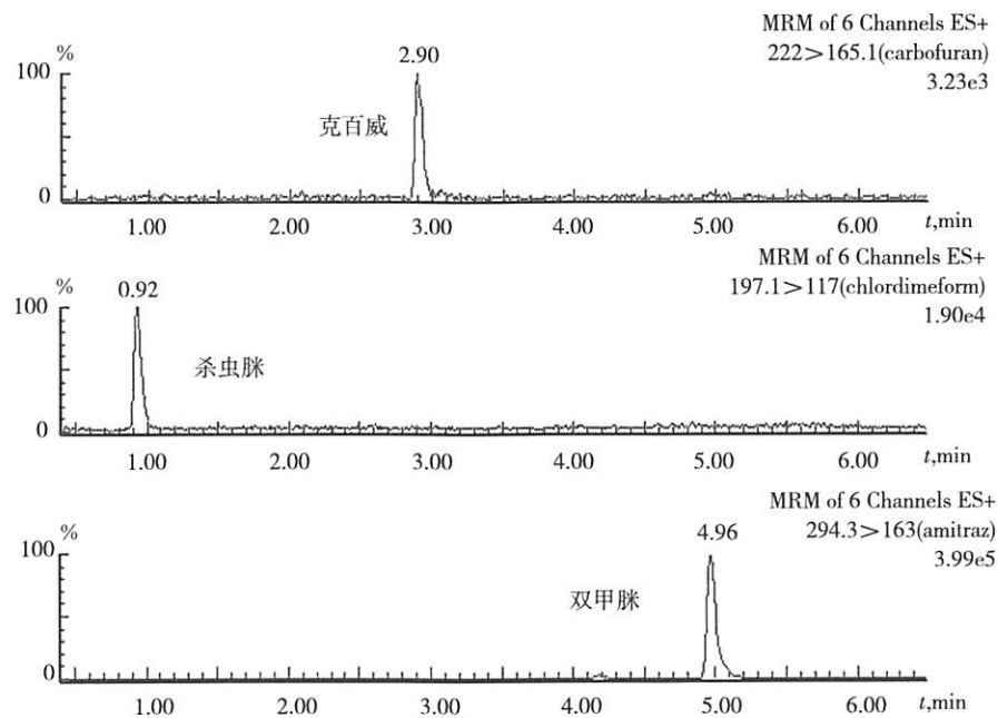
图 A. 1 克百威、杀虫脒和双甲脒基质匹配混合标准溶液(0. 50 μg/L)定量离子色谱图
